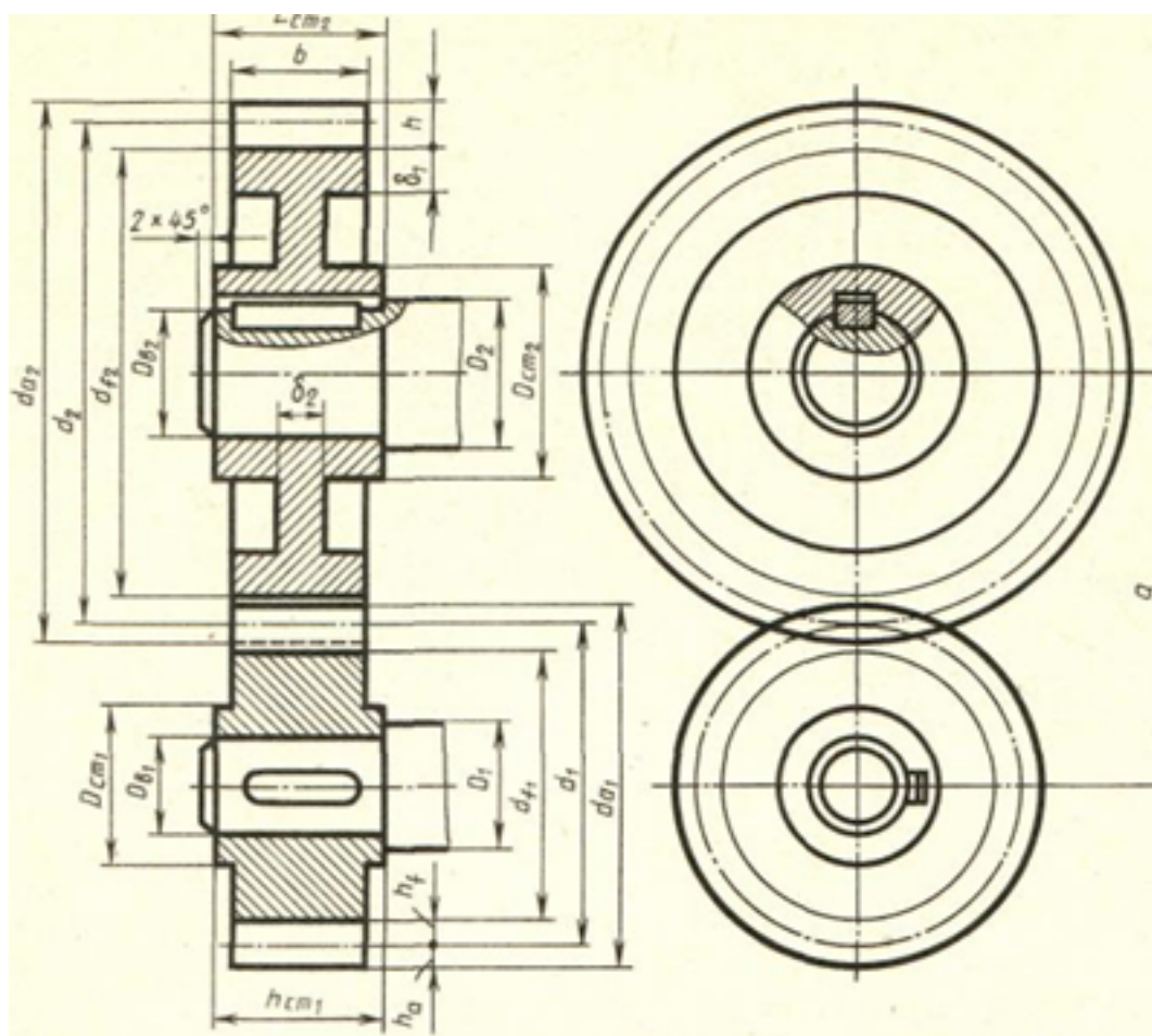
Элементы зубчатого зацепления
