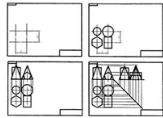
Рис. 2 Построение аксонометрической проекции геометрических тел
