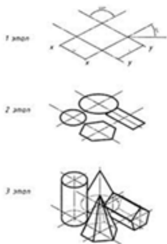
Рис. 2 Построение аксонометрической проекции геометрических тел
