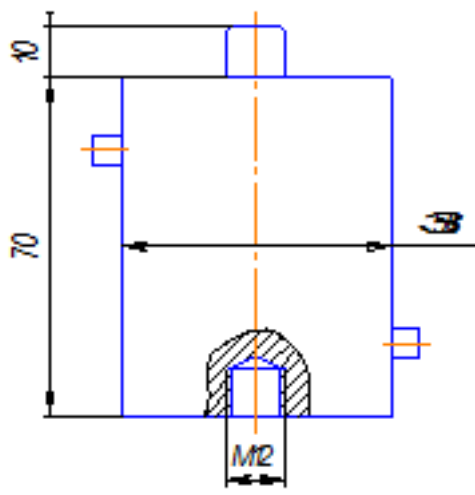
Рисунок 1. Пример гидроцилиндра.
