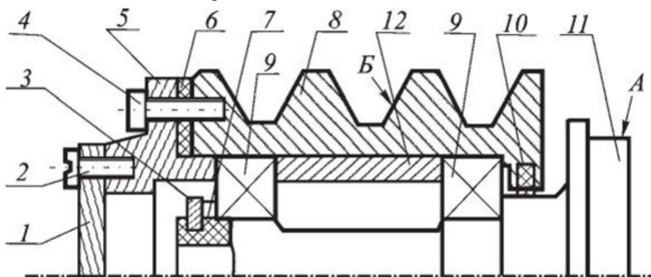
Рисунок 2 - Эскиз сборочной единицы (Сб.11 — Ступица):
