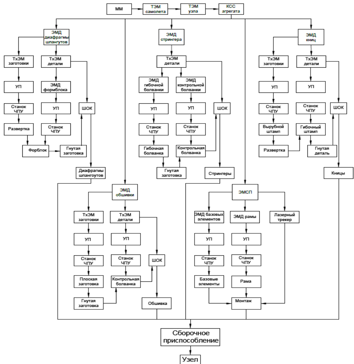
Рисунок 2.____ – Схема увязки и обеспечения взаимозаменяемости (наименование узла)
