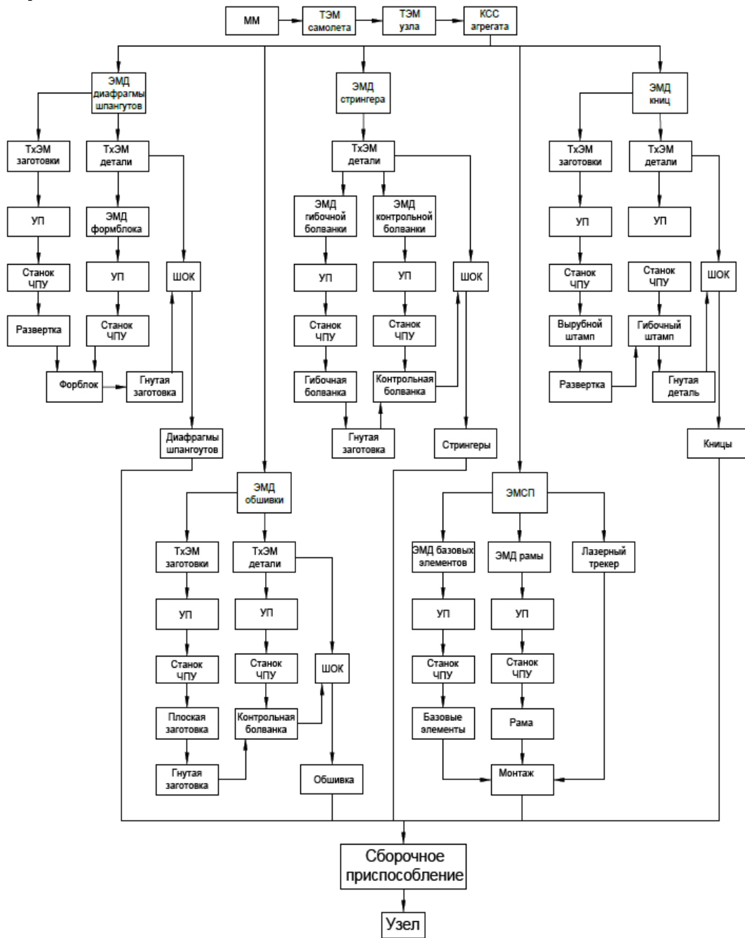
Рисунок 1.2_– Схема увязки и обеспечения взаимозаменяемости(наименование узла)
