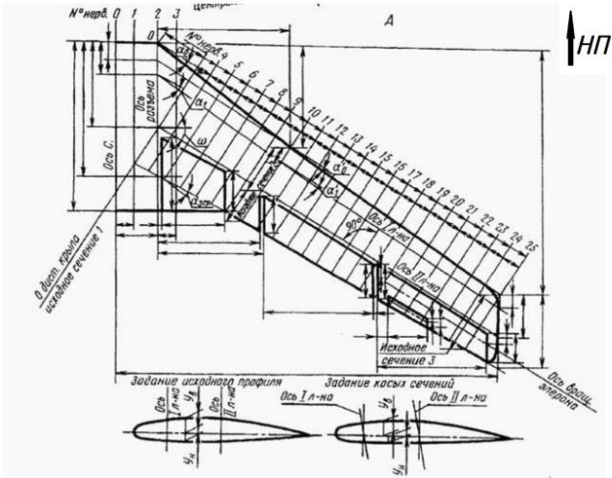
Рисунок 2.4 – Пример расположения основных элементов крыла самолета (из ГОСТ 2.419-68 «Пример выполнения теоретического чертежа крыла самолета»)
