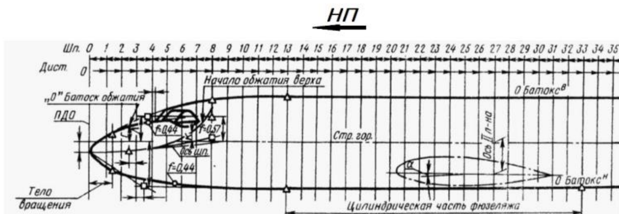
Рисунок 2.3 – Пример расположения основных элементов фюзеляжа самолета (из ГОСТ 2.419-68 «Пример выполнения теоретического чертежа фюзеляжа самолета»)
