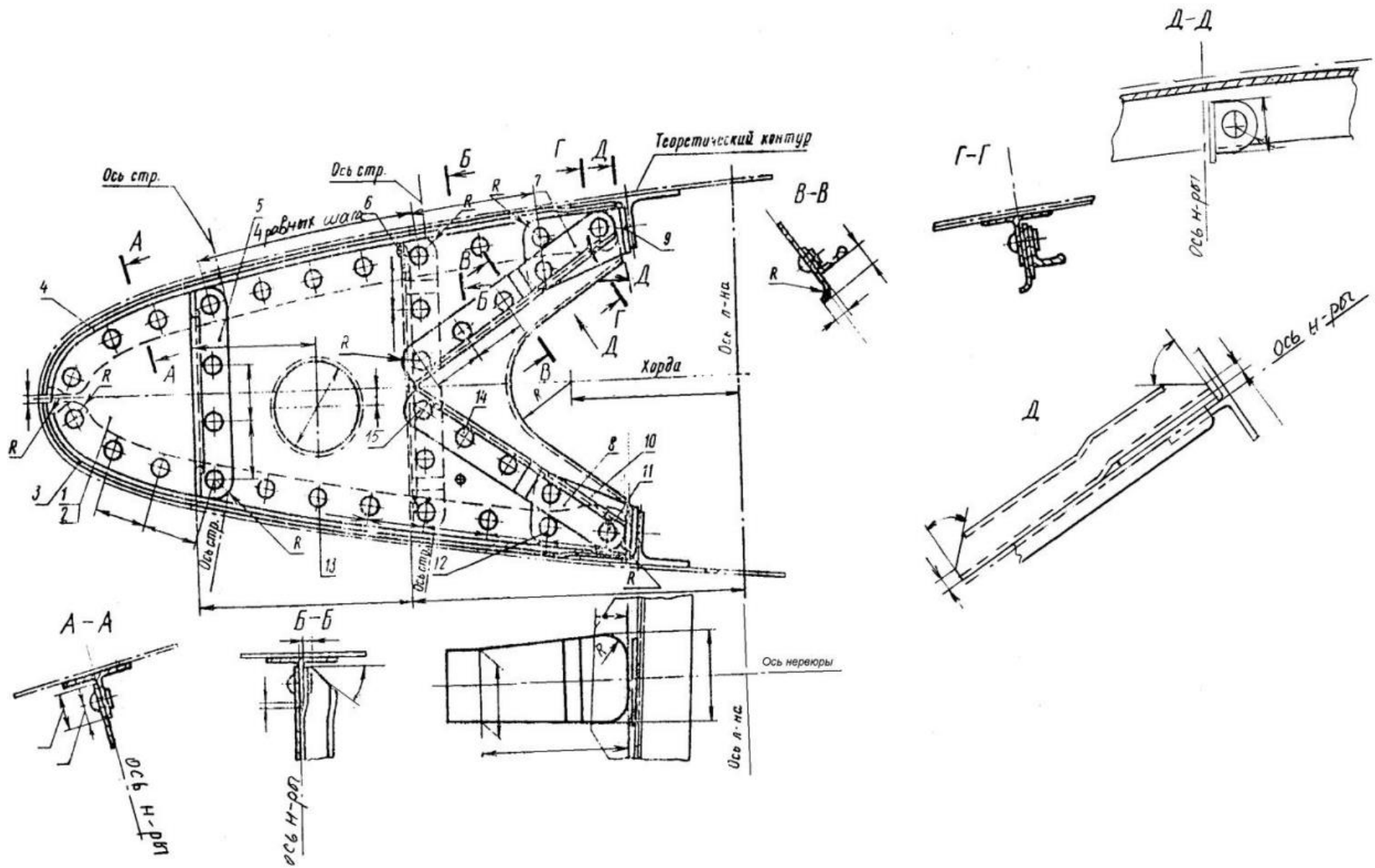
Рисунок 2.5 – Пример выполнения сборочного чертежа носка нервюры (из ГОСТ 2.419-68)
