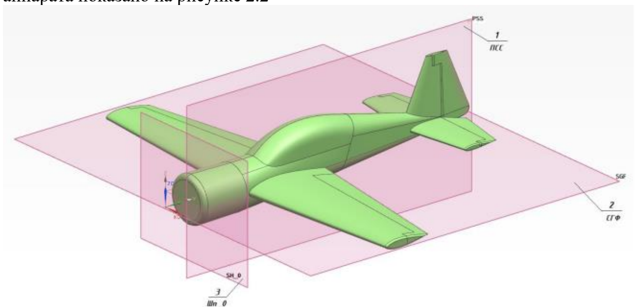
Рисунок 2.2 – Расположение основных координатных плоскостей летательного аппарата
